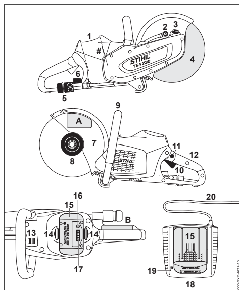
1 Акумулаторна шахта
